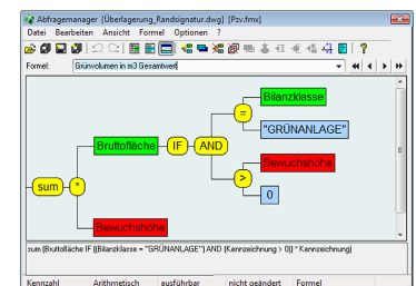
Der Abfrage-Manager von WS LANDCAD
