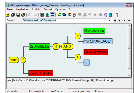
Der Abfrage-Manager von WS LANDCAD
