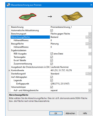
DGM - Volumenkörper aus Massenberechnungen unterstützen BIM
